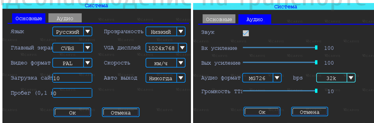
Рисунок 26 – Окно «Система»
