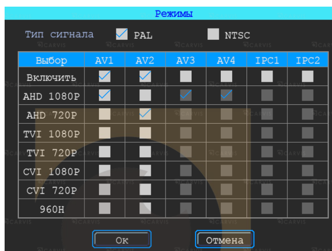
Рисунок 29 – Окно «Режимы»
