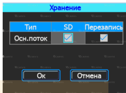
Рисунок 33 – Окно «Хранение»
