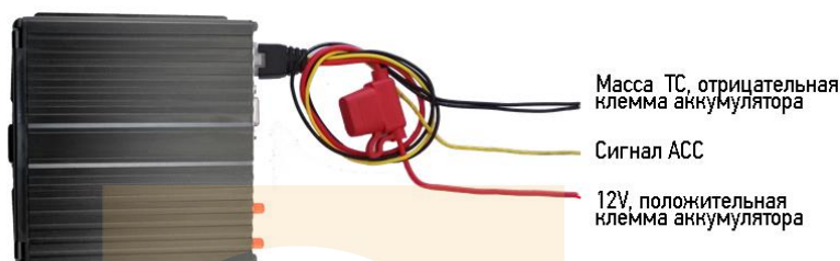
Рисунок 6 – Подключение питания к видеорегистратору
