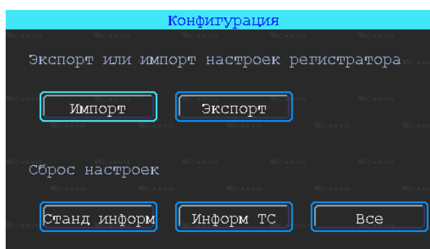
Рисунок 44 – Окно «Конфигурация»
