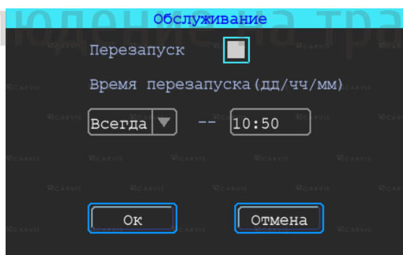
Рисунок 46 – Окно «Обслуживание»
