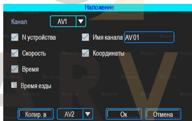
Рисунок 34 – Окно «Наложение»
