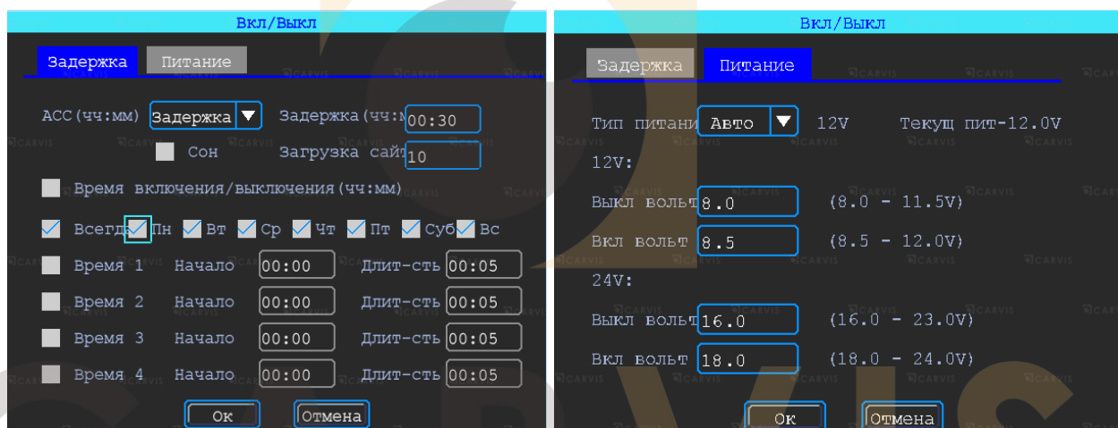
Рисунок 25 – Окно «Вкл/Выкл»
