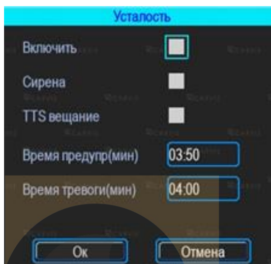
Рисунок 51 – Окно «Усталость»
